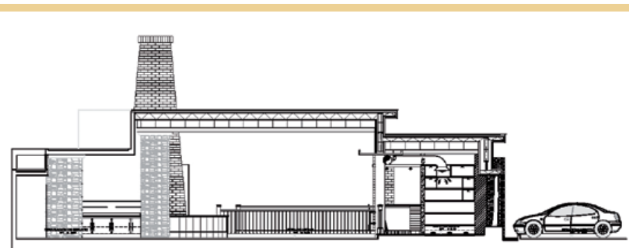
CORTE 2-2
