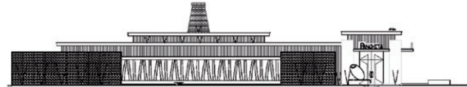
ELEVACION A (Calle Coronel Inca)
