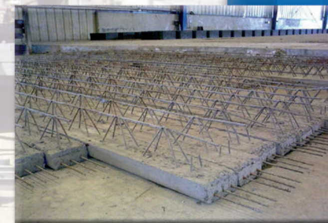
Viguetas de alma abierta Pretensadas
